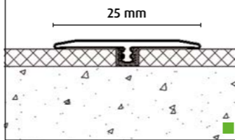
FN fit-fix Nr. 8 4,5-5,5 mm
