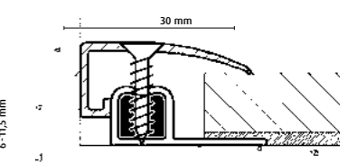
Abschlussprofil 10,5-16 mm
