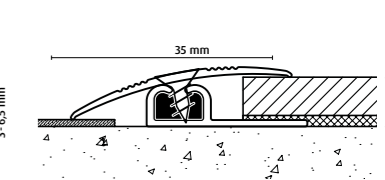
Übergangsprofil 1-10,5 mm
