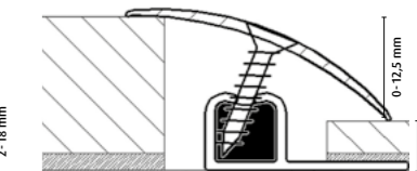
Übergangsprofil 5 - 22,5 mm
