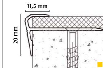
FN fit-fix Nr. 12 5-5,5 mm
