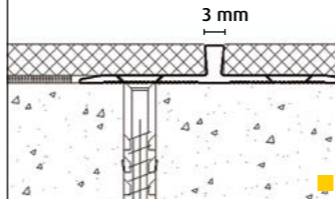
FN simple-fix Nr. 34 >2,5 mm
