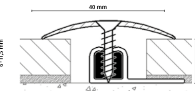
Bewegungsprofil 10,5 - 16 mm
